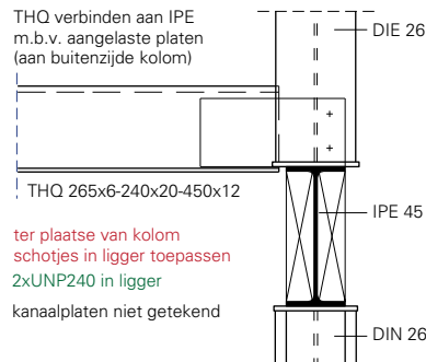
Verbinding windverband (strip en ligger).
