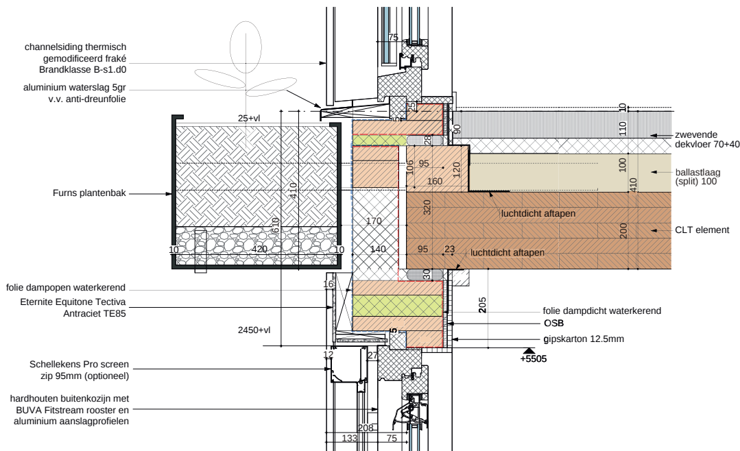
Detail aansluiting CLT vloer op HSB gevel en rondgaande plantenbak.
